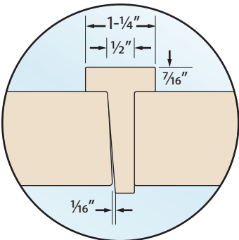
Square T-Astragal
